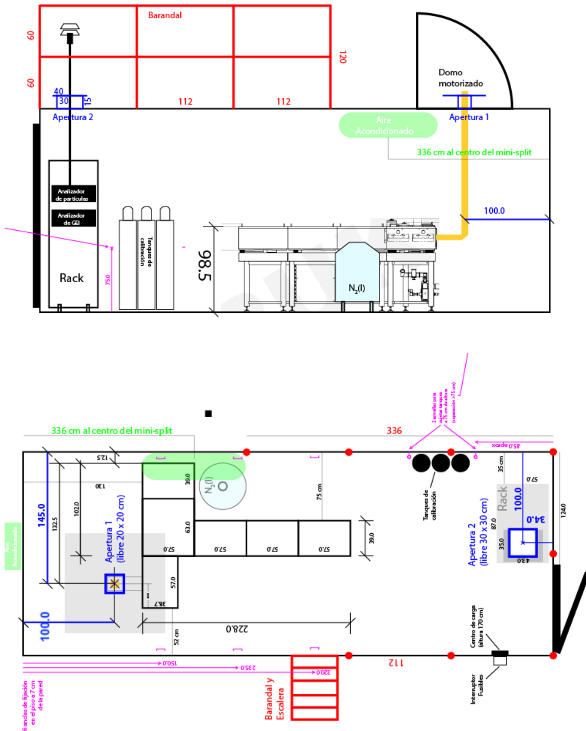
Figura 2. Diseño final de la distribución del instrumento IFS 125/HR en el contenedor vista de lado (panel superior) y vista de arriba (panel inferior).
