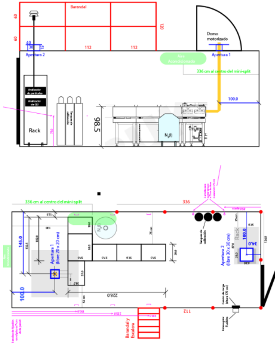
Diseño final de la distribución del instrumento IFS 125/HR en el contenedor
