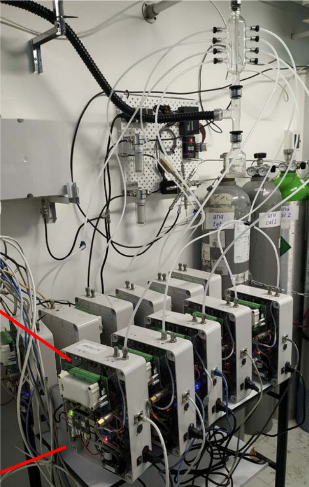
Sensores NDIR de “bajo costo” (Sensair HPP)
