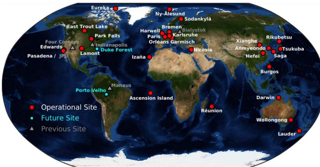
Distribución de estaciones de la red TCCON en el mundo
