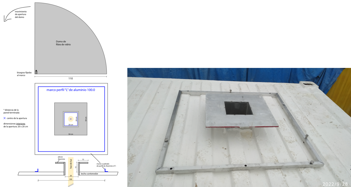
Figura 2. Diseño (izquierda) del domo motorizado que se está construyendo de fibra de vidrio para proteger los componentes ópticos del rastreador solar cuando no se esté usando y fotografía (derecha) de la base que lo alojará.
