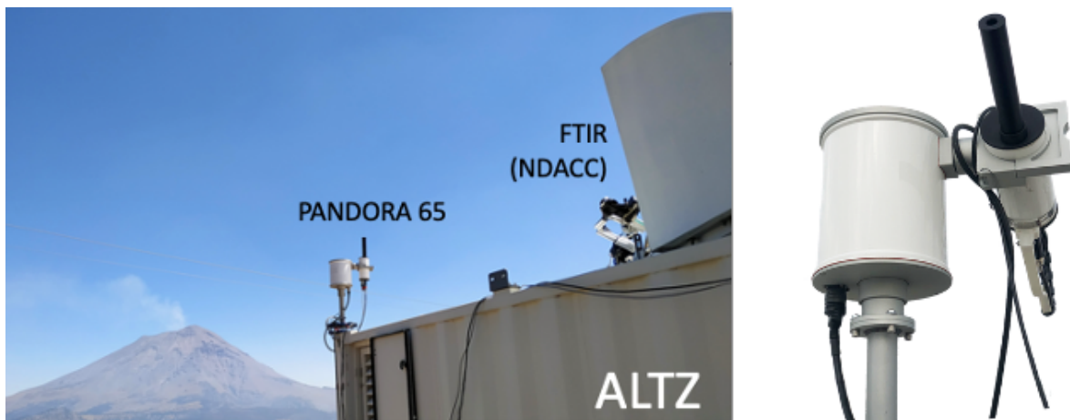
Figura 5. Izq: Fotografía de los sensores remotos Pandora y FTIR que se operan en el observatorio atmosférico de altura en Altzomoni, Parque Nacional Ixta-Popo. Derecha: cabezal de sistema de seguimiento solar del instrumento Pandora.
